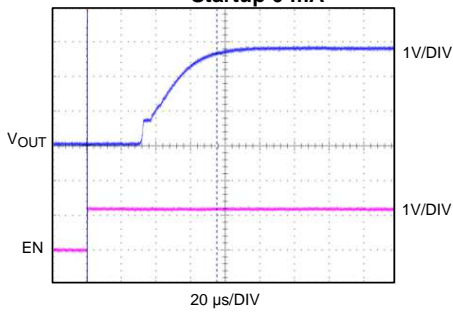
Startup 0 mA
